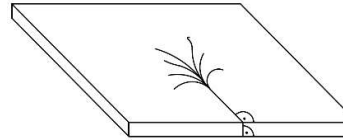
Fissure thermique en palmier
