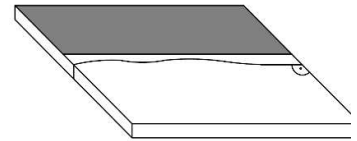
Fissure thermique longitudinale
