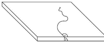
Fissure thermique normale
