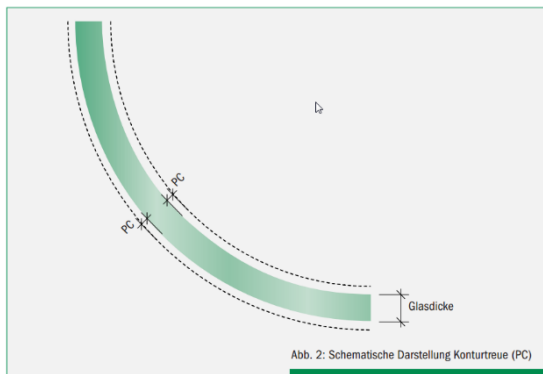
Fig. 2 Représentation schématique de la fidélité des contours/ Glasdicke : épaisseur du verre
