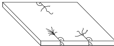
Thermischer Randbruch
