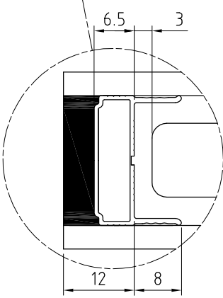
CANALINA RIBASSATA CON GUIDA
