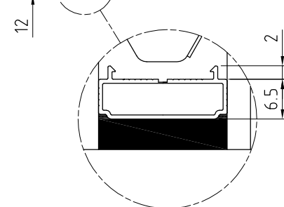
CANALINA RIBASSATA CON INCASTRO
